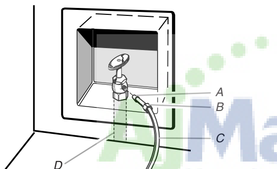
A. Bulbo B. Tuerca C. Tubería de cobre (al refrigerador) D. Línea de suministro doméstica ( \frac{1}{2} " como mínimo)
