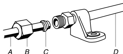
A. Tubería al refrigerador B. Tuerca (comprada) C. Férula (comprada) D. Línea provista del refrigerador
