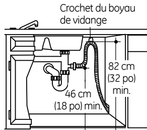
Installation avec raccord en T
