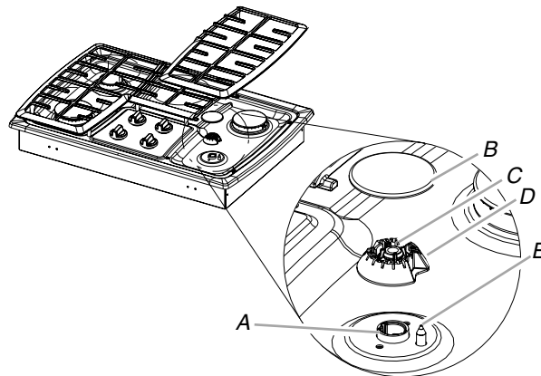
A. Porte-gicleur B. Chapeau du brûleur C. Ouverture du tuyau de gaz D. Base du brûleur E. Électrode d'allumage
