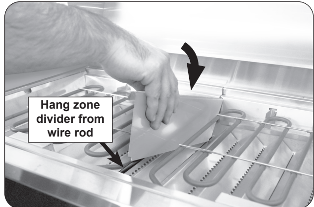
Fig. 25-3 Install zone divider
