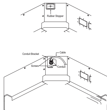
Figure 181: Using a Conduit.
