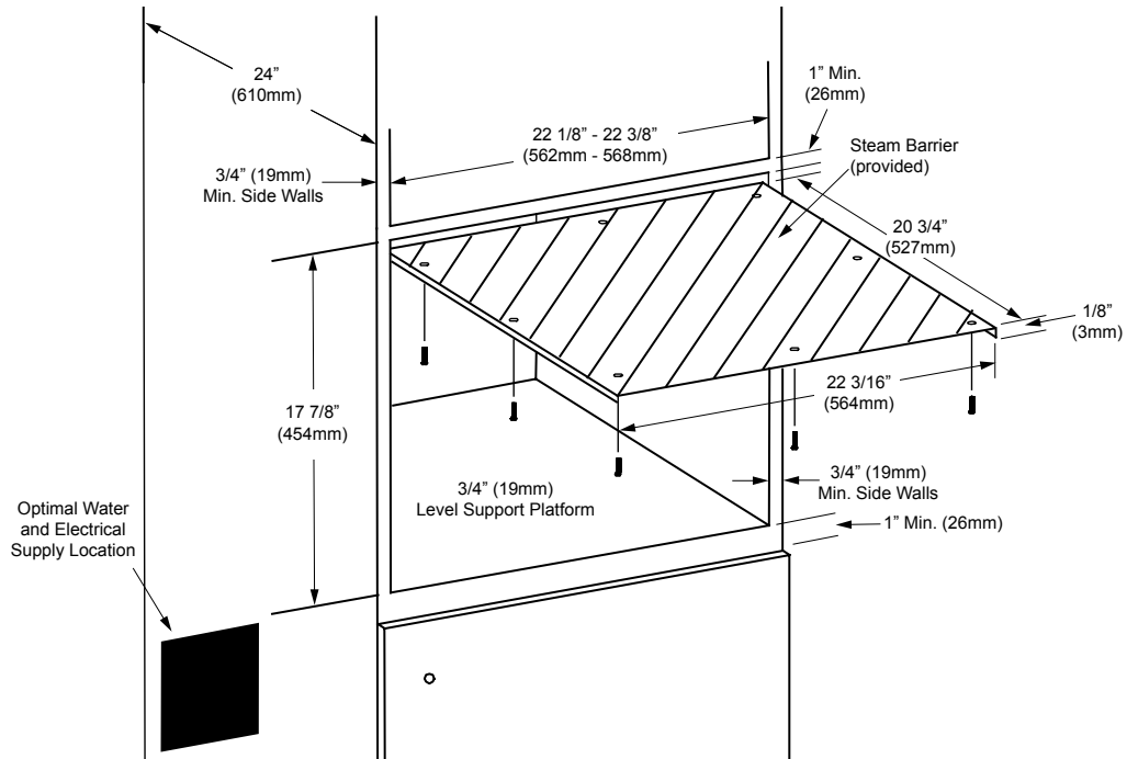
CUTOUT DIMENSIONS
