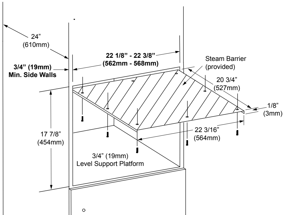
CUTOUT DIMENSIONS
