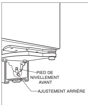
Réglage de la base à roulettes arrière.
