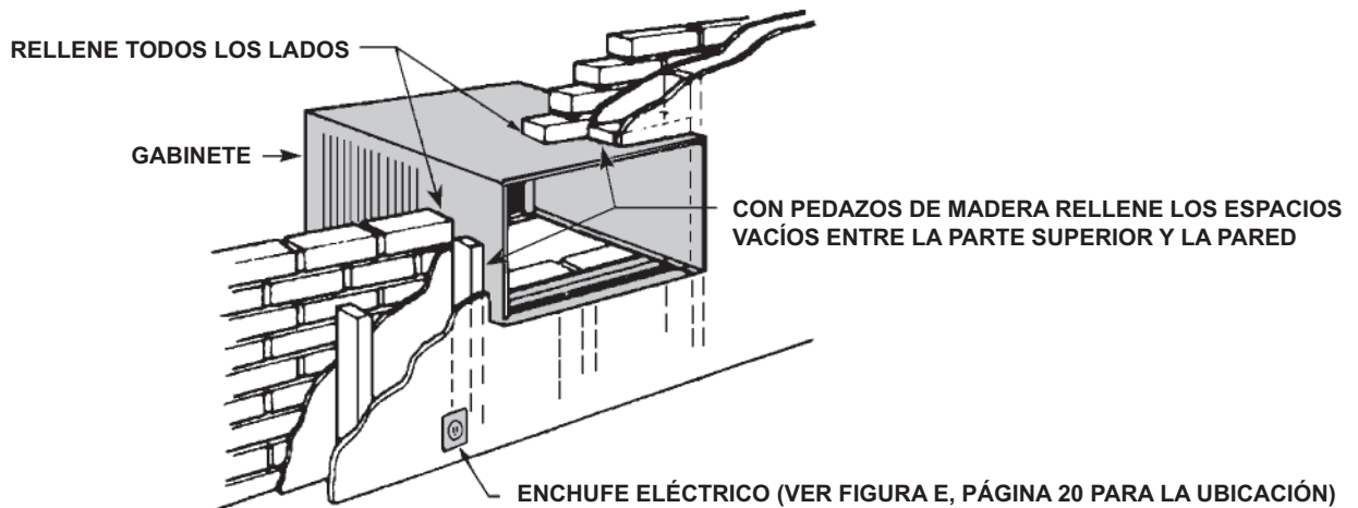
FIGURA D - CONSTRUCCION EN LADRILLO
