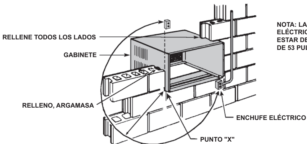
FIGURA E - CONSTRUCCION EN ALBAÑILERÍA SOLIDA
