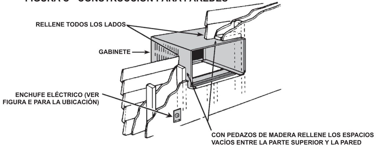
FIGURA C - CONSTRUCCION PARA PAREDES
