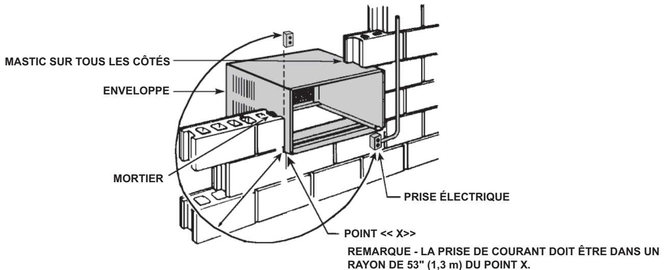
FIGURE E CONSTRUCTION EN MAÇONNERIE SOLIDE
