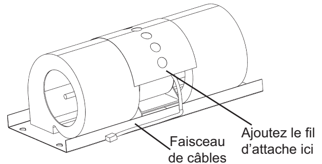
Figure 14 : Vue arrière du ventilateur
