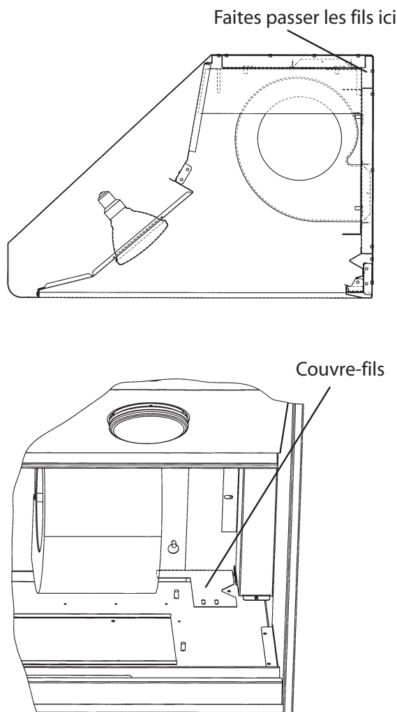
Figure 18 : Débouché horizontal
