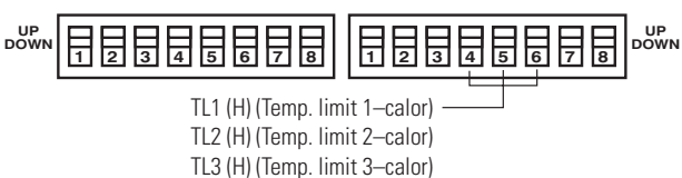
Limitación de temperatura durante el modo HEAT (todas las temperaturas están en °F)
