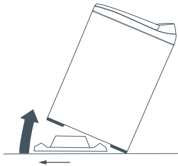
Fig.1 Inclinez la laveuse vers l'arrière pour retirer le support moulé
