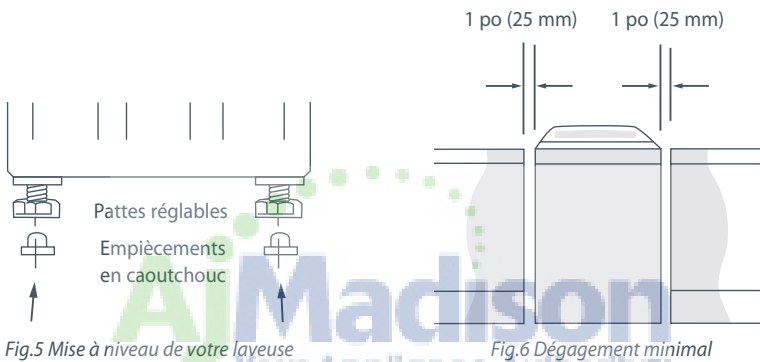
Fig.5 Mise à niveau de votre laveuse
