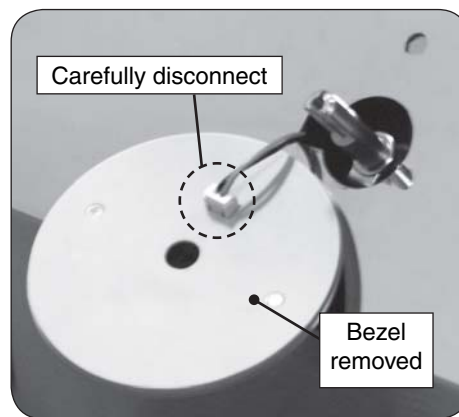
Fig. 16-1 Remove bezel
