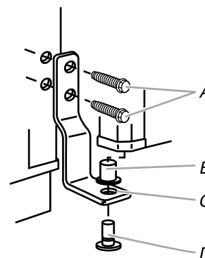
A. Vis de charnière à tête hexagonale B. Douille de l'axe de la charnière C. Charnière D. Axe
