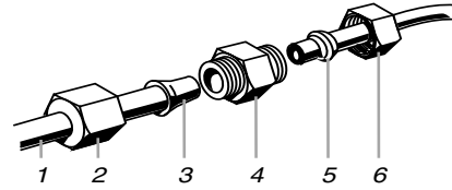
1. Tubería al refrigerador 4. Acoplamiento (adquirido) 2. Tuerca (provista) 5. Férula (adquirida) 3. Bulbo 6. Tuerca (adquirida)
